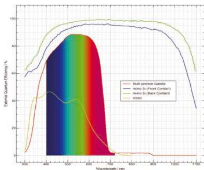
Badanie charakterystyk ogniw PV i reakcji widmowej
