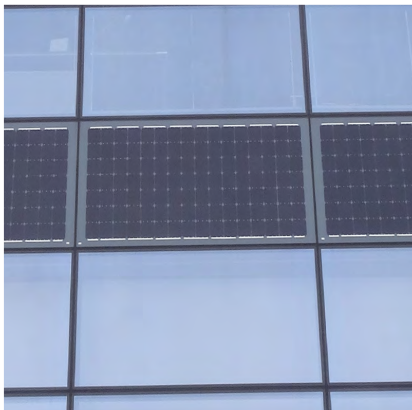
Produkty ML System: Spandrele ściany osłonowej BIPV moduły nieprzeźierne w technologii szkło-szkło
