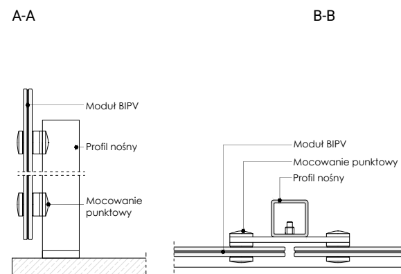
BALUSTRADA MOCOWANA PUNKTOWO
